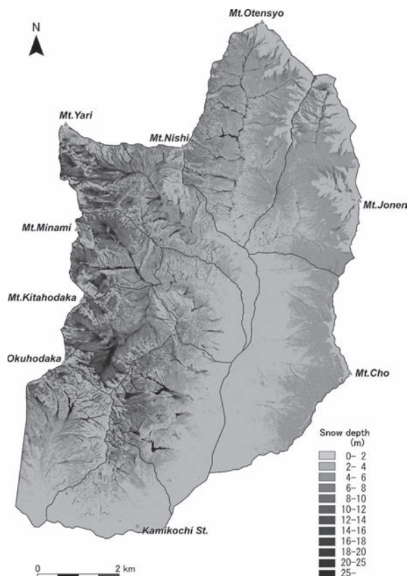
図10. 航空レーザ測量による上高地梓川流域における積雪深分布（鈴木・佐々木，2012）
