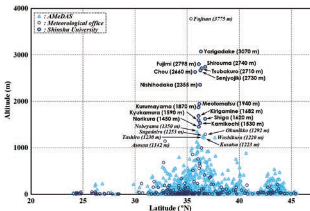
図8. 気象庁による気温観測地点と信州大学による気象観測地点の緯度と標高の関係。
