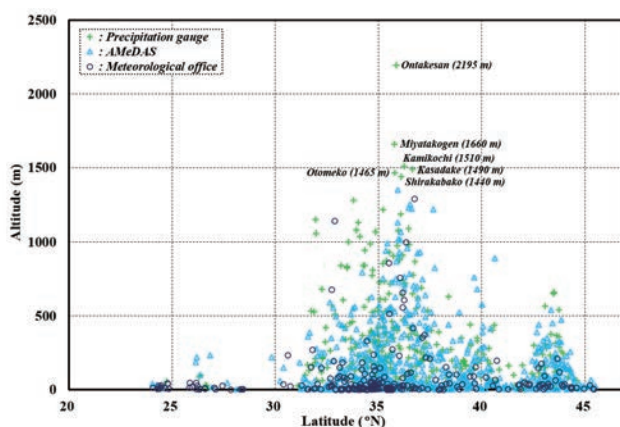
図4. 気象庁による降水量観測地点の緯度と標高の関係。
